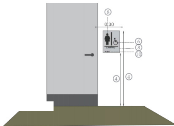
Figura GE 06 - 1 Ubicación de señal en puerta
